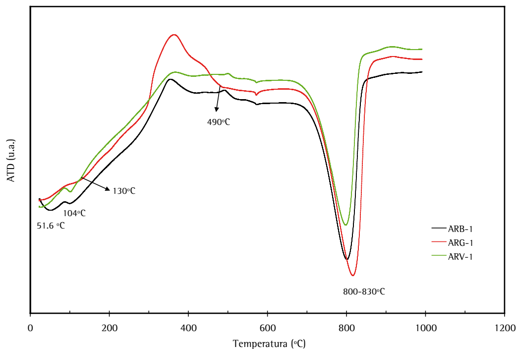
Figura 9. Evolución de los ATD obre muestras de árido reciclado mixto.
