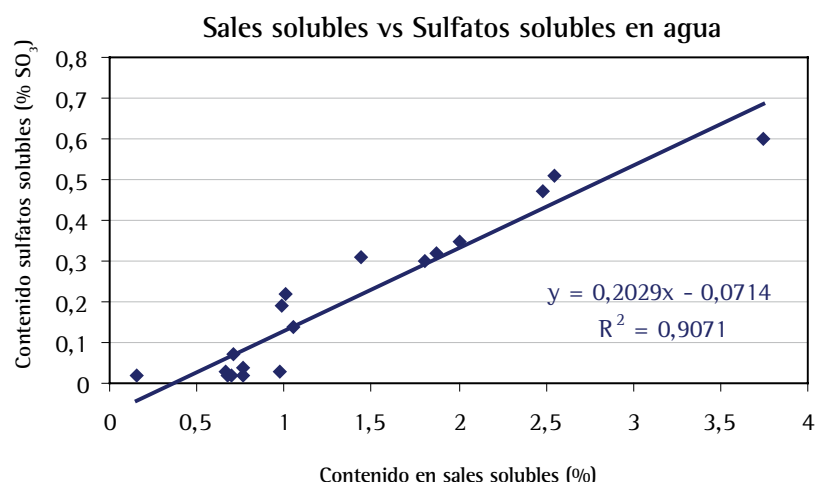
Figura 13. Relación entre sales solubles y sulfatos solubles en agua.
