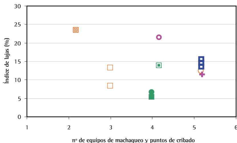
Figura 27. Influencia del número total de equipos de machaqueo más puntos de cribado en el índice de lajas del árido reciclado.
