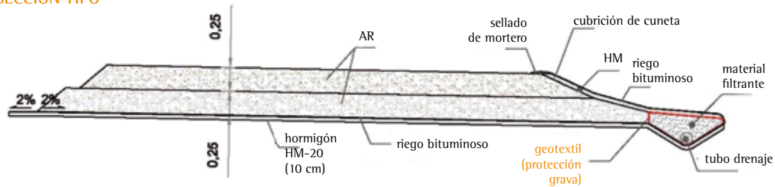
Figura 16. Sección tipo del tramo de prueba de la Orkonera.
