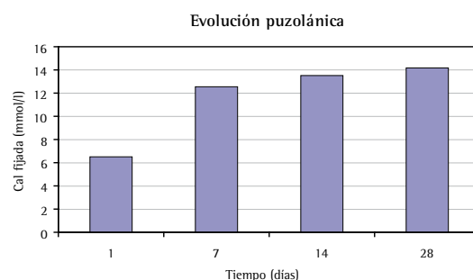
Figura 5. Actividad puzolánica de cerámico reciclado finamente molido: 2ª muestra.
